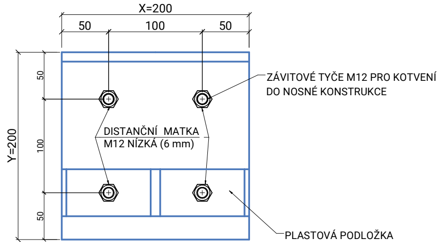
POHLED ZADNÍ
