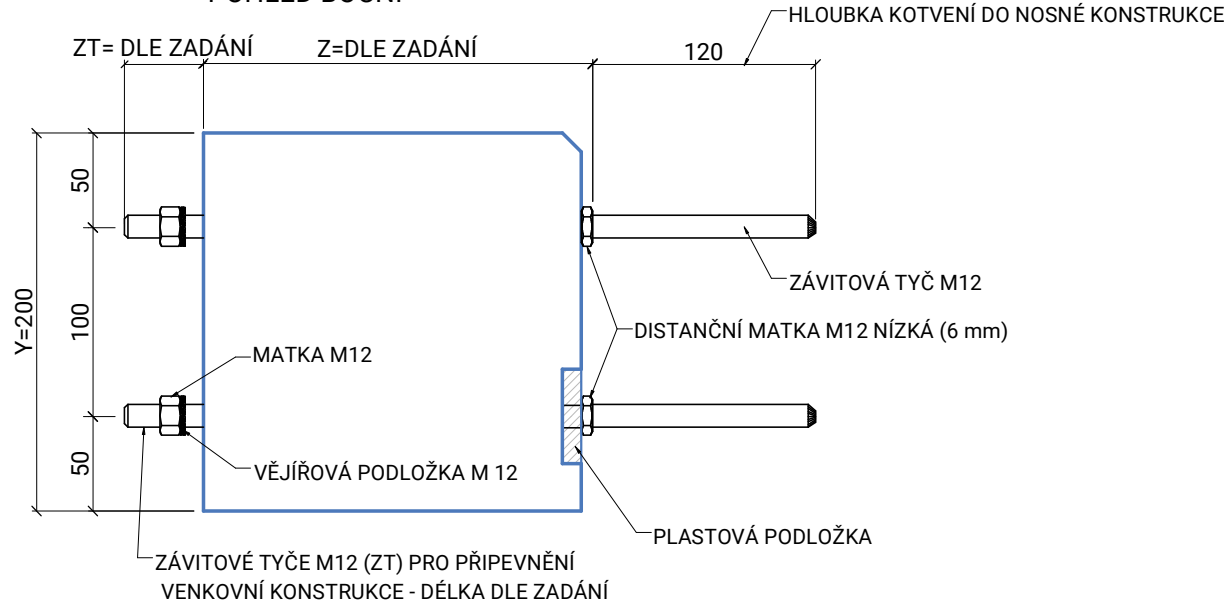
POHLED BOČNÍ
