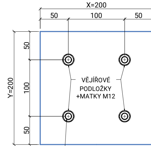
POHLED PŘEDNÍ
