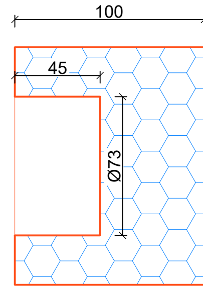
ŘEZ BLOKEM
